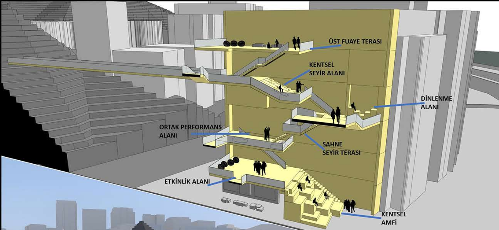
BB KESİTİ
