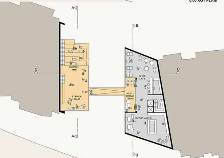
+5.00 KOT PLANI
